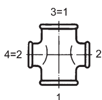
1 schéma 1/D
